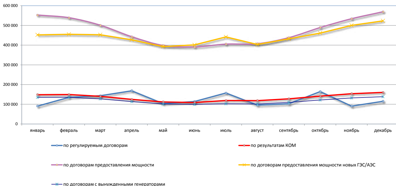
Рис. 4.14. Цены покупки мощности с ОРЭМ в 2012 году
