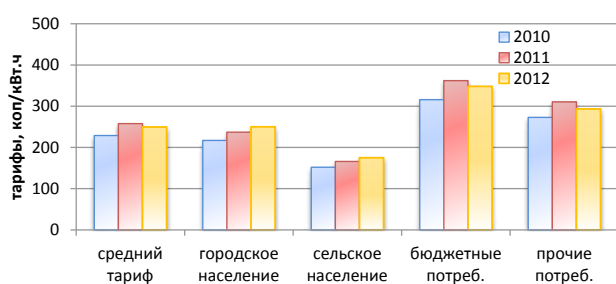
Рис. 4.9. Динамика изменения тарифов и цен на электрическую энергию для потребителей ОАО «Мордовская энергосбытовая компания» за 2010-2012 гг. (по каждой категории потребителей приведены средние тарифы (цены) на электрическую энергию)
