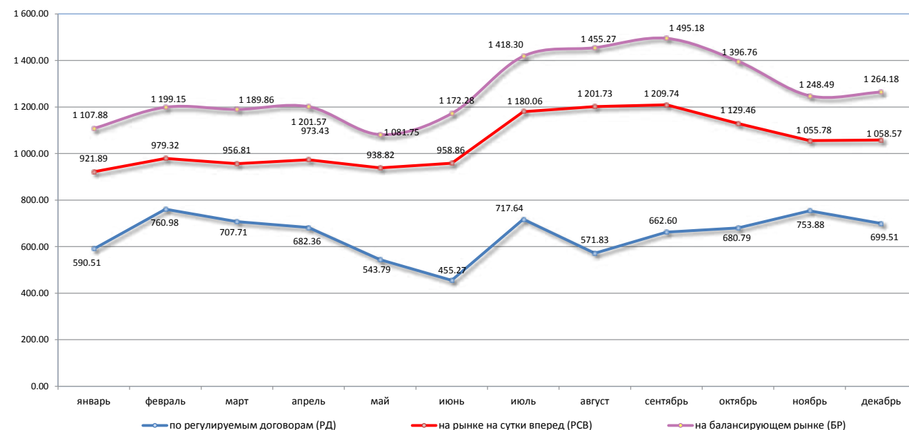
Рис. 4.10. Цены на покупку электрической энергии на ОРЭМ в 2012 году (руб./МВт.ч.)
