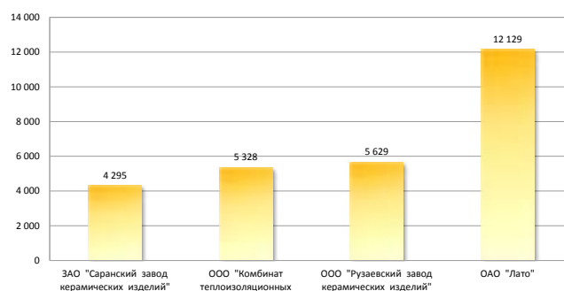
Рис. 4.20. Энергоёмкие предприятия отрасли «Промышленность строительных материалов» (тыс.кВт.ч.)
